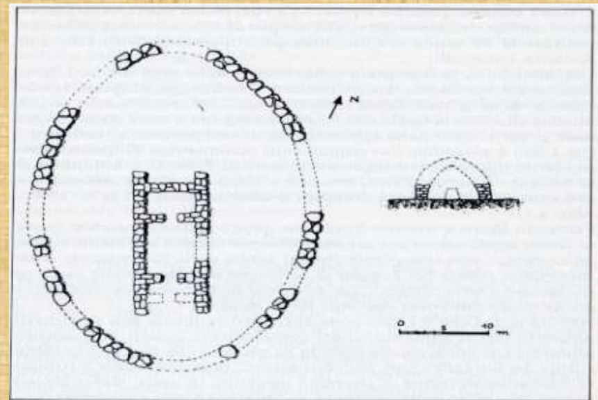
Planimetria e sezione dell'edificio megalitico «a megaron» di Domu 'e Ursia
